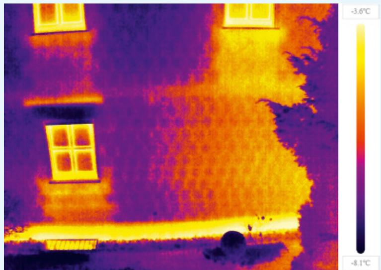
Helle Stellen in der Thermographie-Aufnahme deuten auf unzureichende Isolierung an Sockel, Heizkörpernische, Fenster und Rollläden hin.
